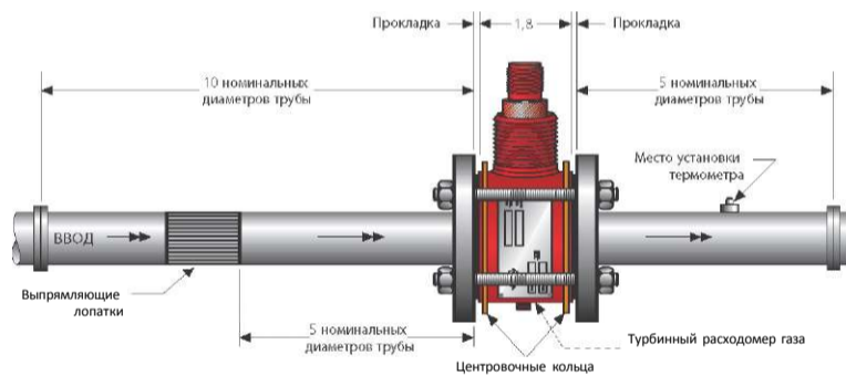
Схема монтажа
