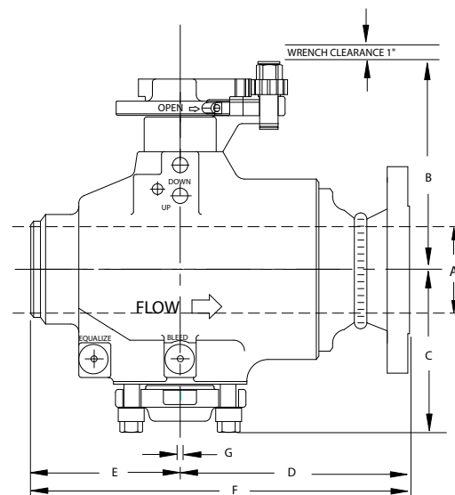
FLANGEWELD TYPE
