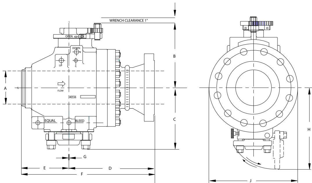
FLANGEWELD TYPE
